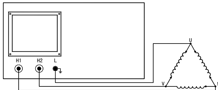
图 3-3 Δ (角) 接法
