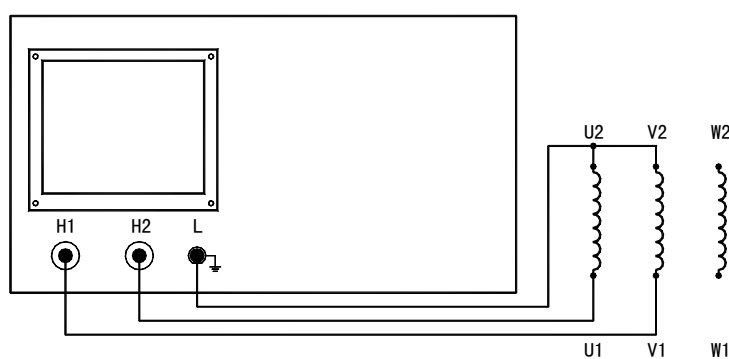
图 3-1 Φ (相) 接法
