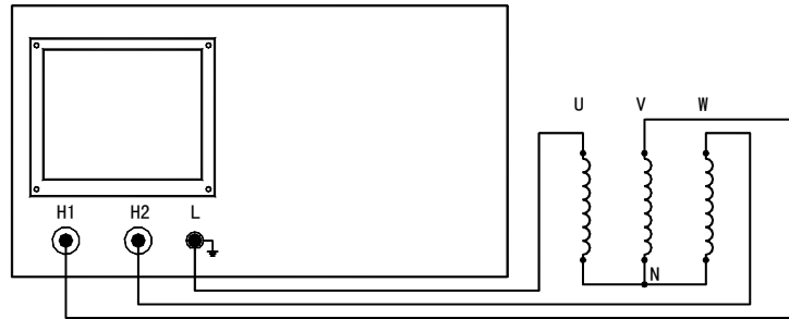
图 3-2 Y (线) 接法
