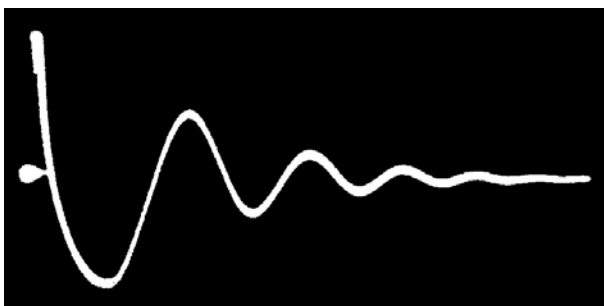
图 3-4 正常波形
